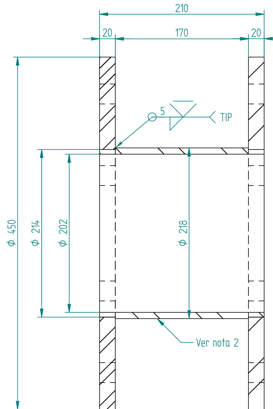
CORTE A-A
